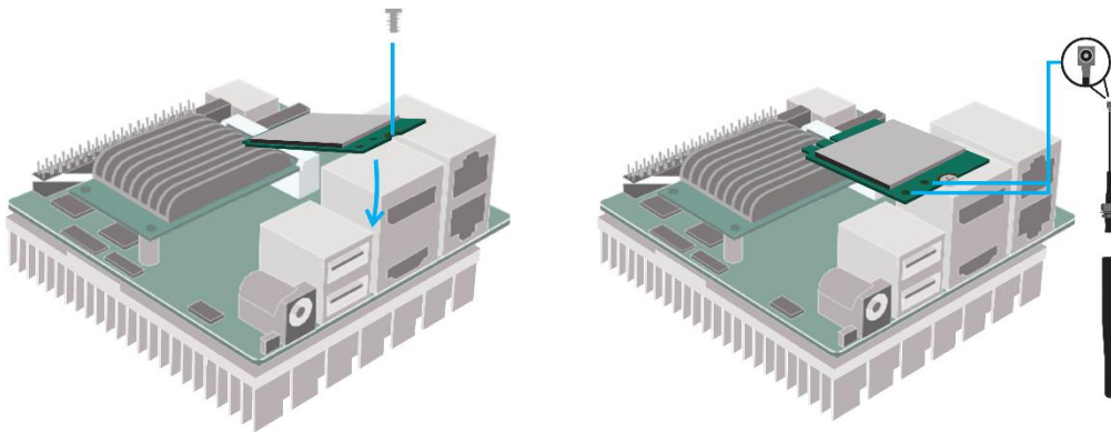
WiFi Module & antennas
